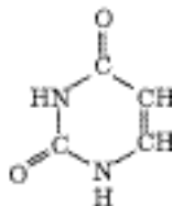
Uracil (RNA)
