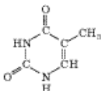
Thymine (DNA)
